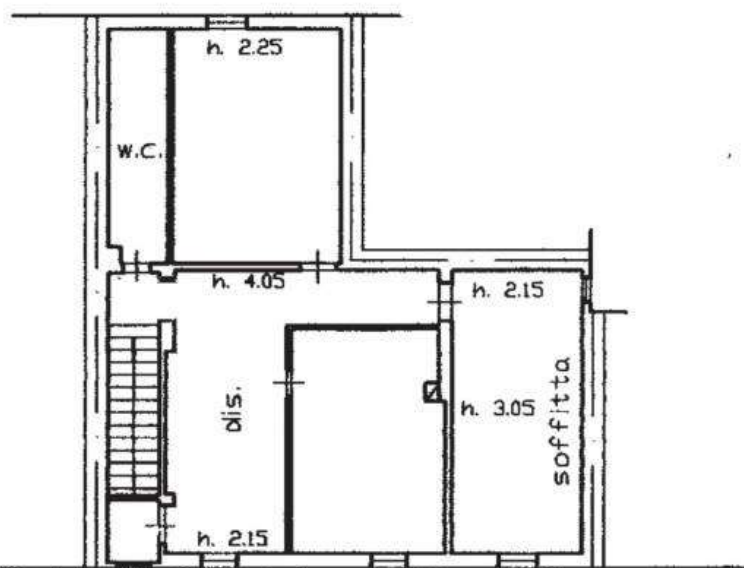
Piano Secondo
